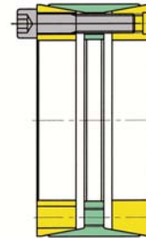
DOBIKON 1015 + Rheinbraun- Spannsatz
