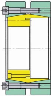
DOBIKON 2019
