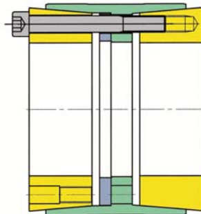
DOBIKON 1013
